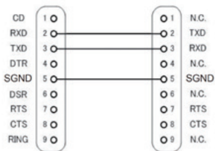
コンピュータCOMポート (Dサブ 9ピンコネクタ)
